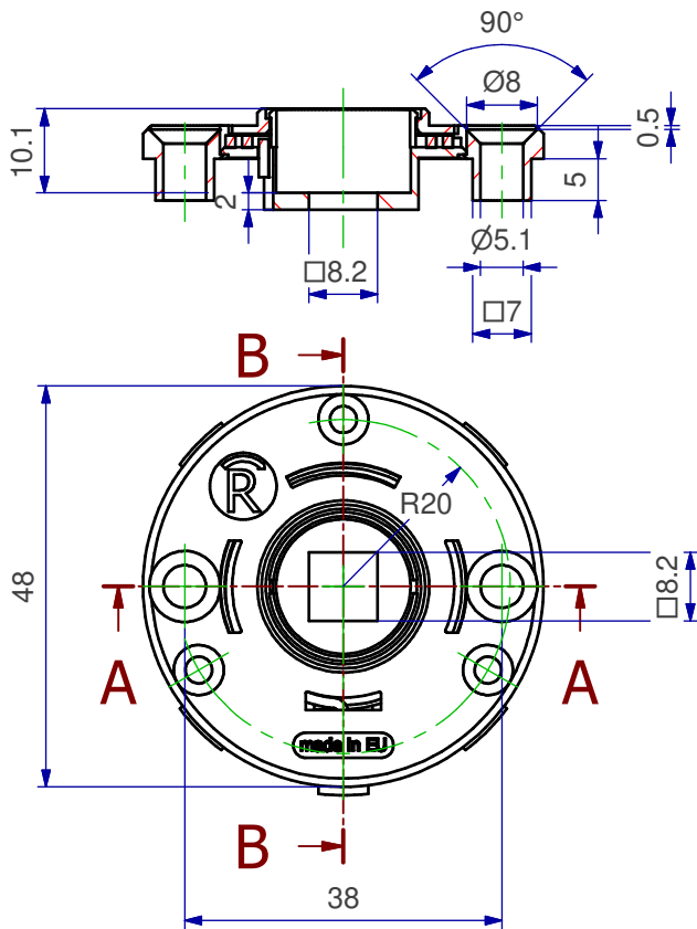
A-A (1:1)
