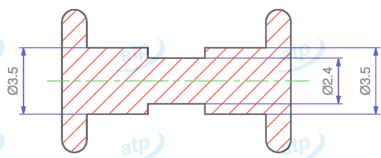
A-A (5 : 1)
